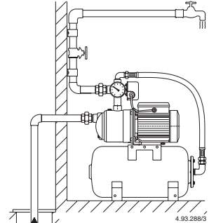
Fig. 2 Funzionamento in aspirazione Suction lift operation Saugbetrieb Fonctionnement en aspiration Funcionamiento en aspiración Sugande funkcion Zuigsituatie Θέση λειτουργίας με κάβητη αναρρόφηση Работа выше уровня жидкости 负吸水头工作
